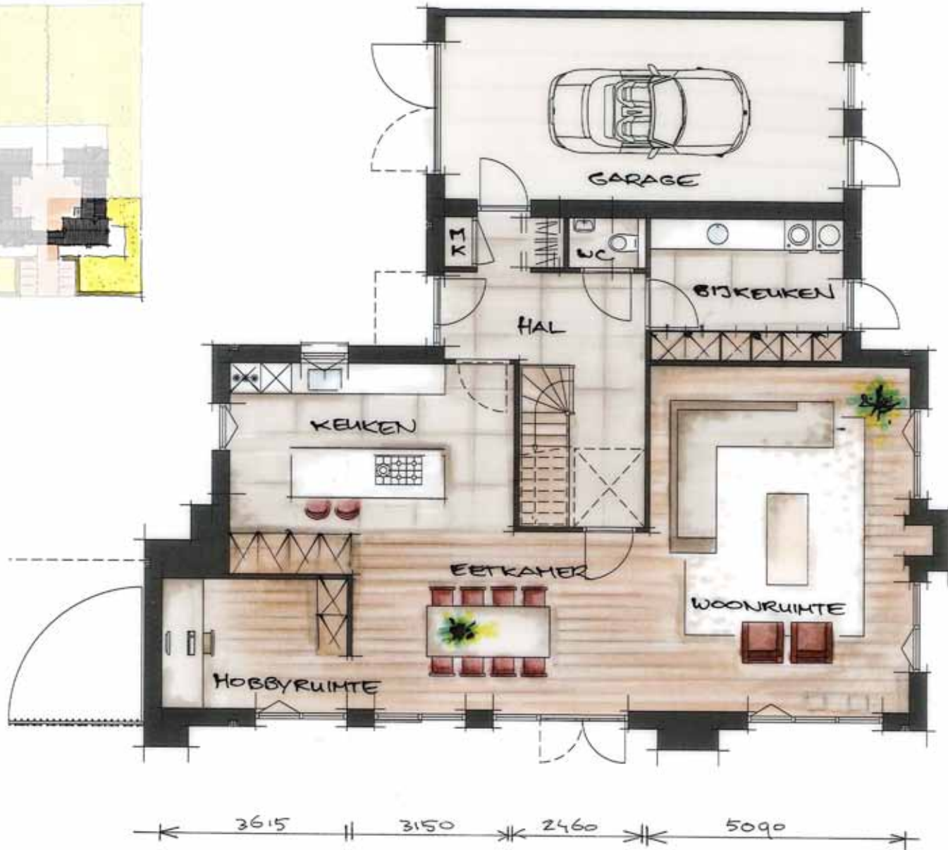
BEGANE GROND
