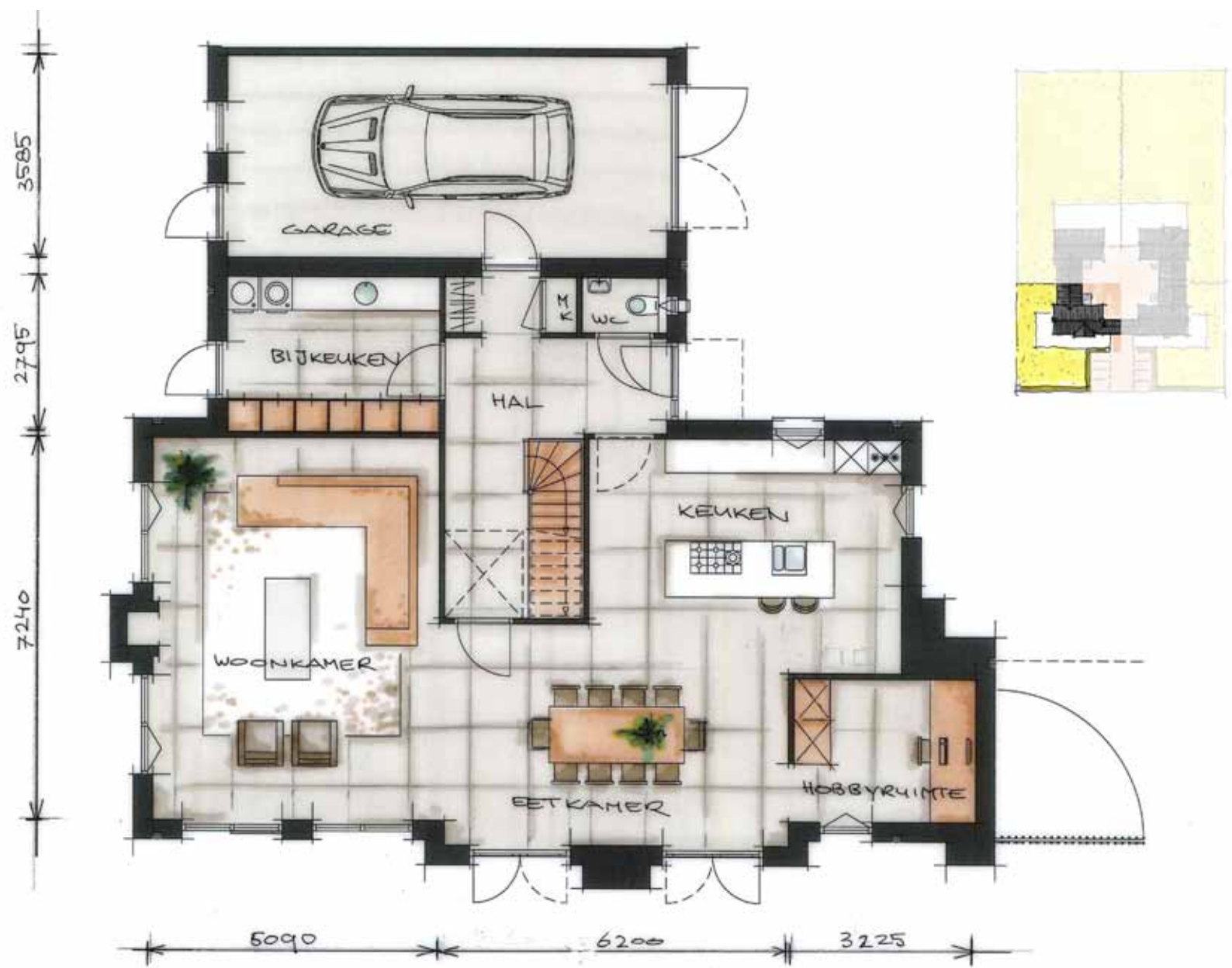
BEGANE GROND
